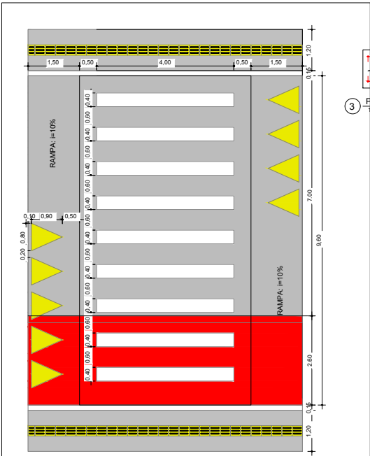
1 DET. PASSAGEM ELEVADA
