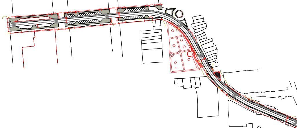
① TRECHO 01 - GEOMÉTRICO 1 : 1000
