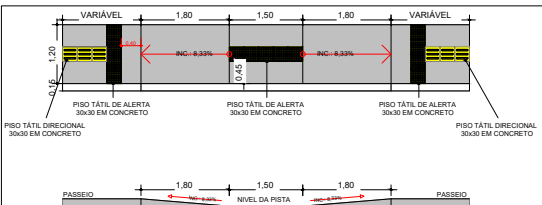
2 DETALHAMENTO RAMPA
