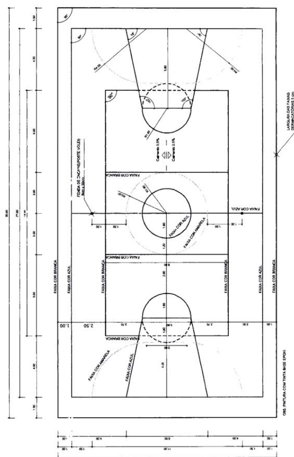
PINTURA DO PISO DA QUADRA - FAIXAS ESCALA 1:100
