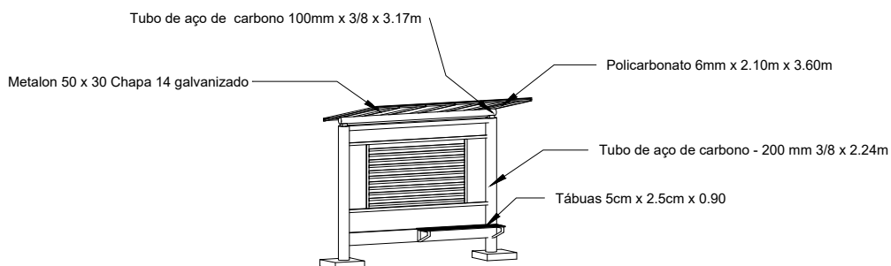
② PROJETO PONTO DE ONIBUS
