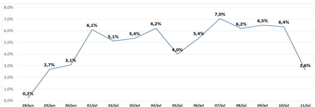
Figura 05. Taxa de progressão da COVID-19 do dia 28/06/2020 a 11/07/2020, Jequié-BA. 2020.
