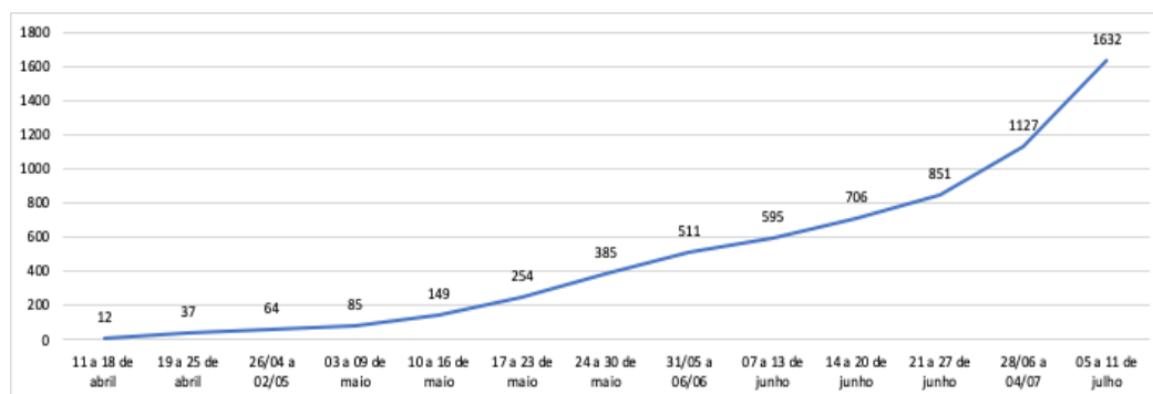
Figura 01. Distribuição do acumulado de casos confirmados por COVID 19 por data de confirmação laboratorial. Jequié-BA 11/04/2020 a 11/07/2020.
