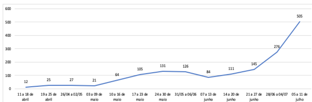
Figura 02. Distribuição dos novos casos confirmados por COVID-19 por semana de confirmação laboratorial. Jequié-BA 11/04/2020 a 11/07/2020.
