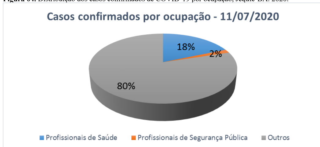
Figura 04. Distribuição dos casos confirmados de COVID-19 por ocupação, Jequié-BA. 2020.
