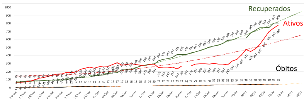
Figura 06. Evolução dos casos ativos, recuperados e óbitos da COVID 19 em Jequié-BA. 2020.
