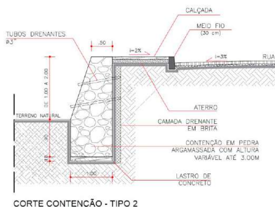
CORTE CONTENÇÃO - TIPO 2
