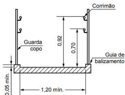
Figura 1 – GUIA DE BALIZAMENTO E GUARDA-CORPO
