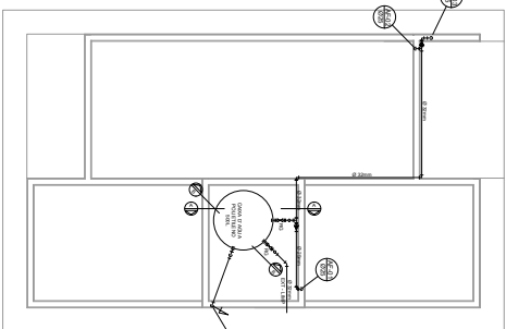
PROJETO HIDRAULICO - BARRILETTA
