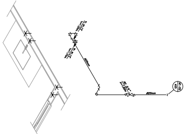
DETALHE ISOMETRICO - 02
