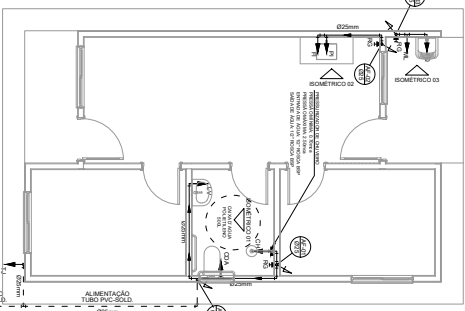
PROJETO HIDRAULICO - PLANTA BAIXA
