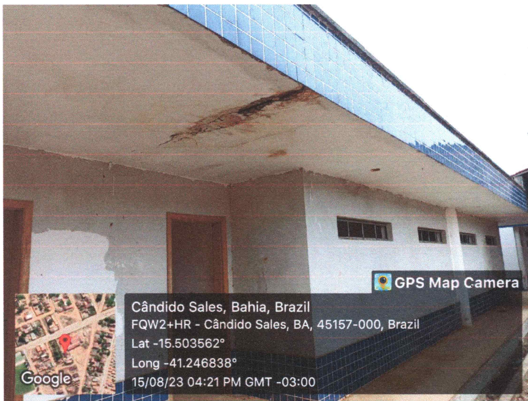
Patologia causada pela infiltração de água entre as salas da creche I e creche II
