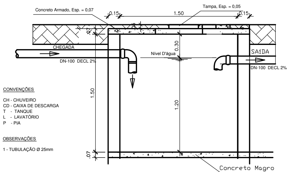
FOSSA SÉPTICA
