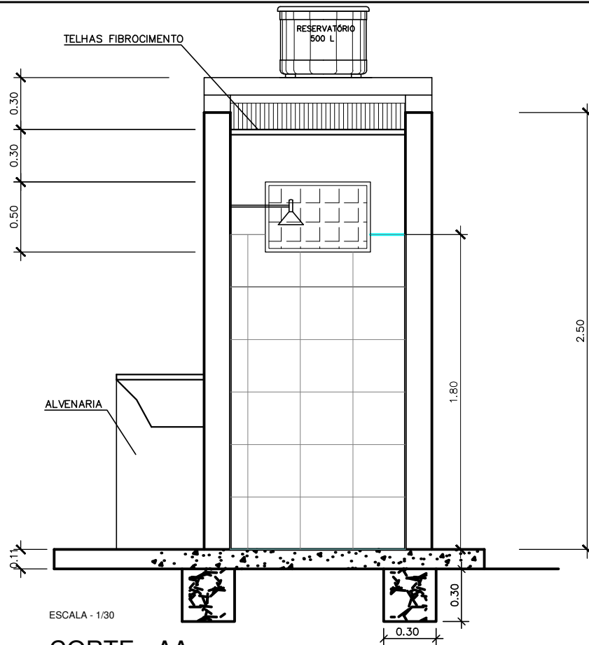
CORTE - AA
