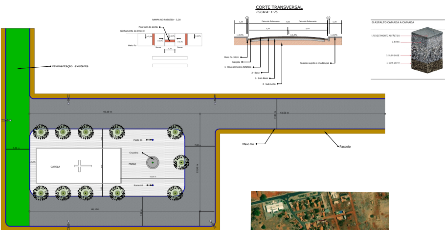
PLANTA BAIXA - PAVIMENTAÇÃO ESCALA: 1:200
